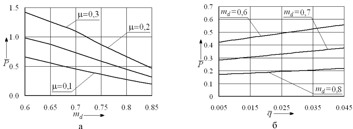
Рис. 2. Зависимости изменения \bar{P} от m_d (а) и \bar{q} (б) для алюминиевого сплава АМг6: а – q = 5 МПа; б – \mu = 0,05
