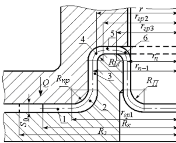
Рис. 1. Схема реверсивной вытяжки осесимметричных деталей с фланцем
